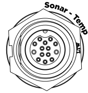
SOLIX port sonar-température
