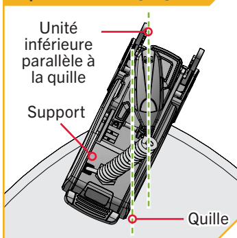
Correction du décalage de la quille à bâbord [-X°]
