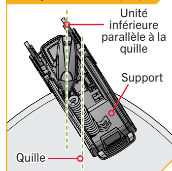
Correction du décalage de la quille à tribord [+X°]
