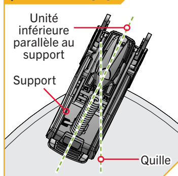
Décalage zéro de la quille à bâbord [0°]
